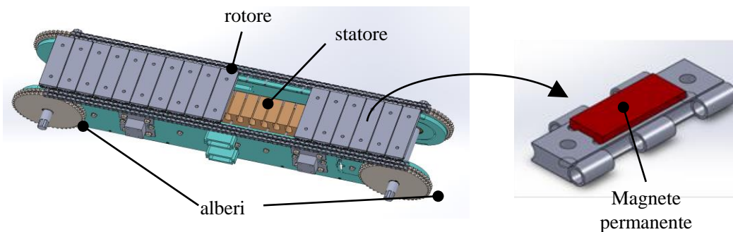
Fig. 2. Rendering di prototipo di motore elettrico rotativo lineare a magneti permanenti superficiali ed avvolgimento statorico concentrato a cave frazionarie.
