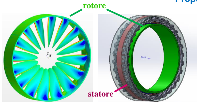
Fig. 1. Rendering dell'elica, con pale montate sulla superficie interna del rotore.
