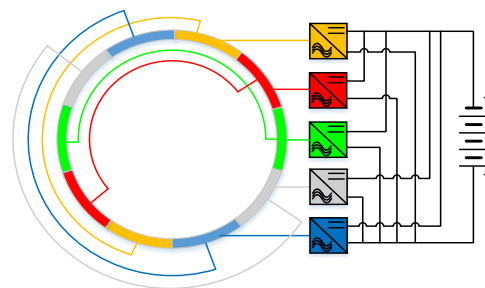
Fig. 4. Segmentazione dello statore in moduli alimentati indipendentemente da più convertitori elettronici connessi al medesimo pacco batterie.
