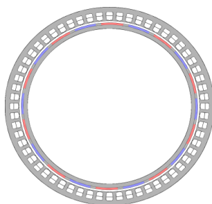
Fig. 3. Sezione trasversale del "rim motor" a magneti permanenti con rotore a struttura "inset permanent magnet".
